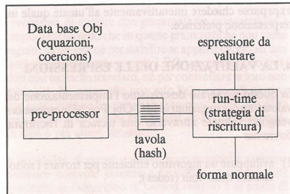
Fig. 3 Implementazione del valutatore di espressioni
