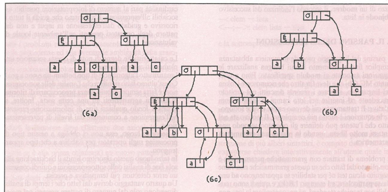
Fig. 2 Rappresentazioni ad albero di espressioni
